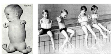
\alpha -苯胺茂二酰亚胺 (反应停)
