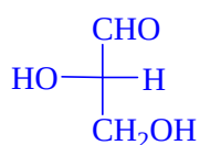
L-(-)-甘油醛
