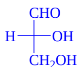
D-(+)-甘油醛
